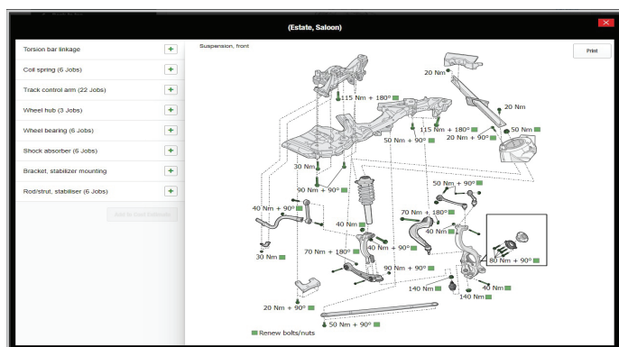
Tekniske tegninger med integrerede tilspændingsmomenter
