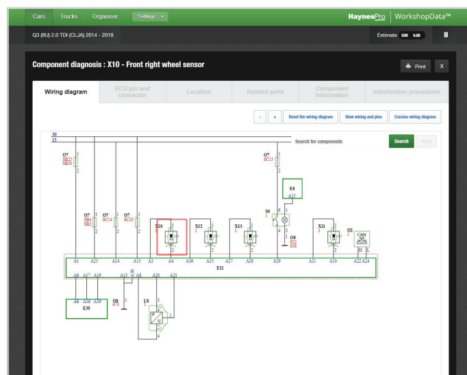
NYHED Komplette elektroniske ledningsdiagrammer
